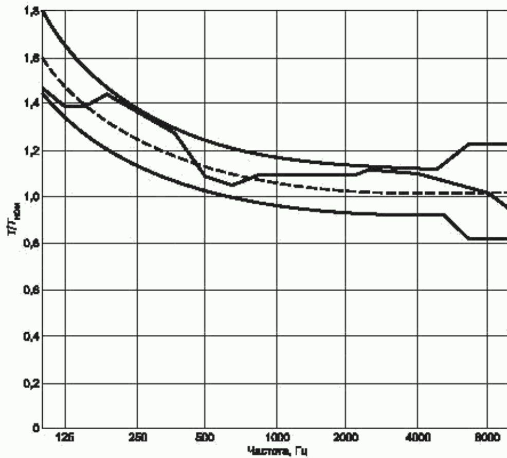
Рисунок Б.4 — Предельные кривые для отношения времени реверберации T к номинальному времени реверберации T_{ном} для камеры объемом 70 \text{ м}^3
