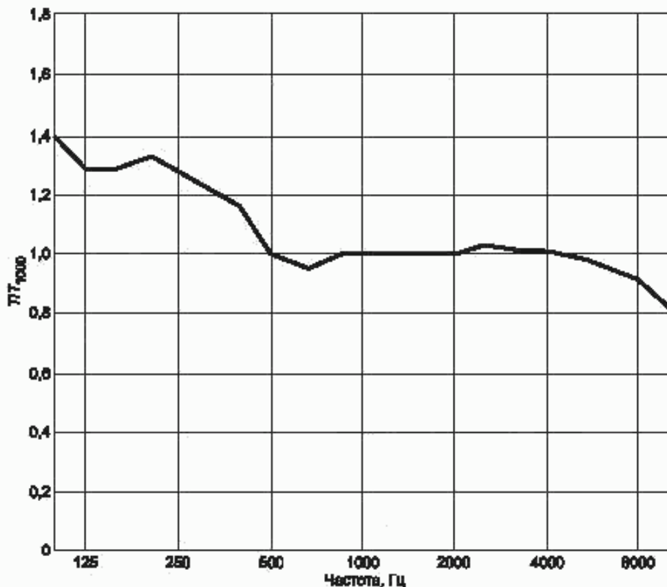
Рисунок Б.5 — График определенного экспериментальным путем времени реверберации (нормализованного по T_{1000} ) в функции среднегогеометрической частоты октавной полосы
