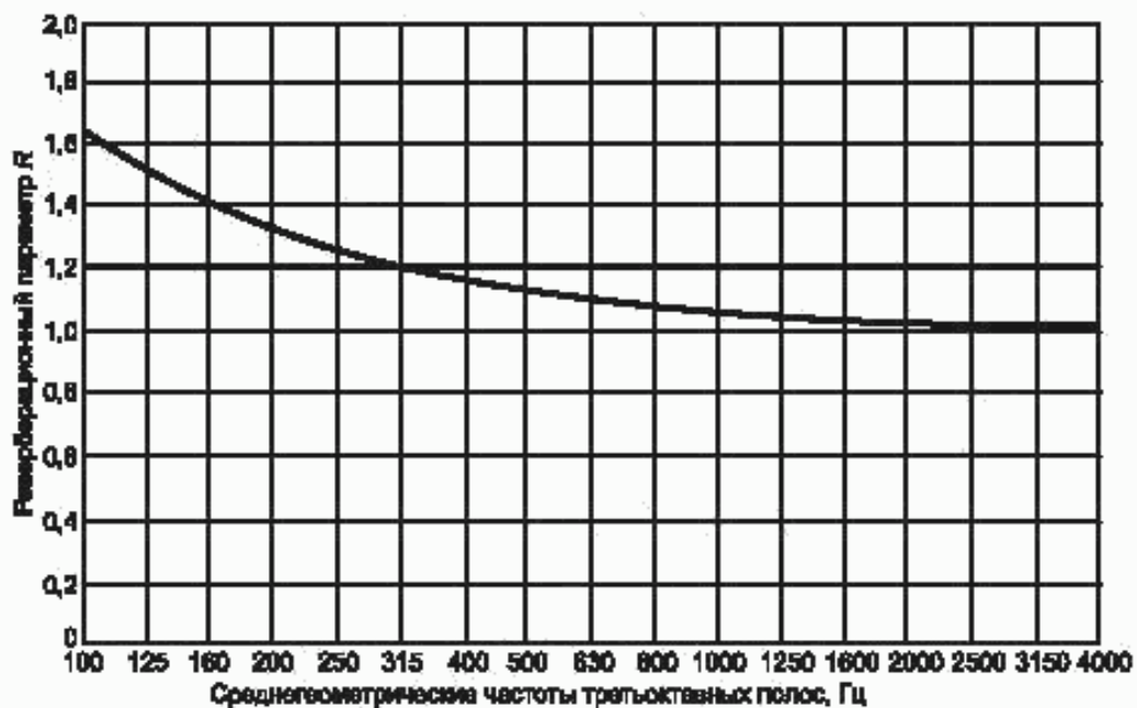
Рисунок Б.3 — Значение реверберационного параметра R для камеры объемом 70 \text{ м}^3 в функции среднегометрической частоты третьоктавной полосы
