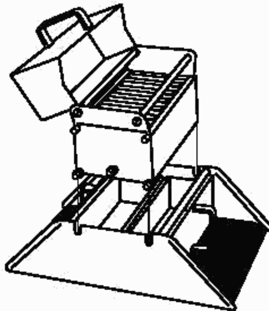
Рисунок А.2 — Множественно-щелевой делитель с системой сортировки
