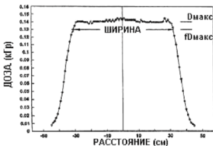
Рисунок 2 – Пример измеренного распределения дозы облучения электронным пучком по ширине пучка, где ширина пучка определена по некоторой заданной доле f от средней максимальной дозы D_{\text{max}}
