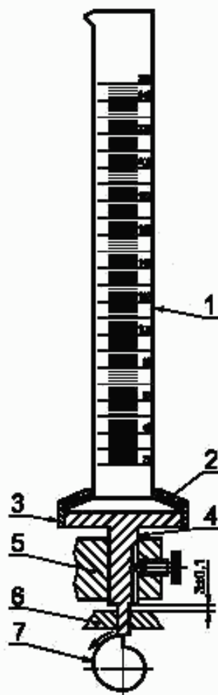
1 — мерный цилиндр; 2 — резиновая итулка; 3 — держатель для мерного цилиндра; 4 — ось; 5 — итулка; 6 — наковальня; 7 — кулачок
