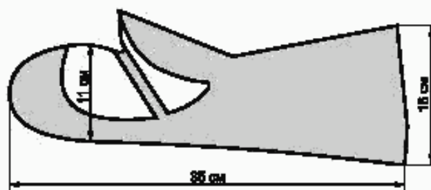
Рисунок 2 — Внутренние минимальные размеры ЗАЩИТНЫХ РУКАВИЦ
