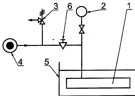
1 — испытуемый СК; 2 — манометр; 3 — предохранительный клапан; 4 — пневматический источник давления; 5 — бак горячей воды; 6 — запорный вентиль
