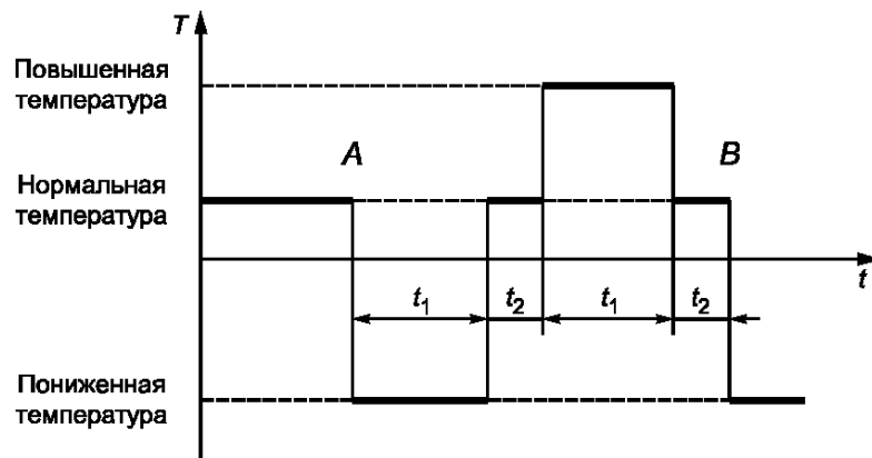
Рисунок 1 — График испытательного цикла
