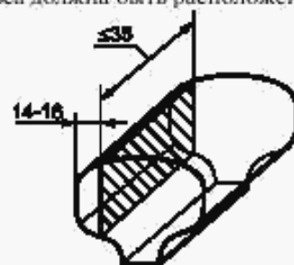
Рисунок 3 — Схема вырезки микрошлифа
