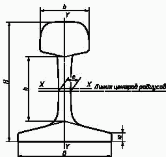
Рисунок 1 — Основные размеры поперечного сечения рельса
