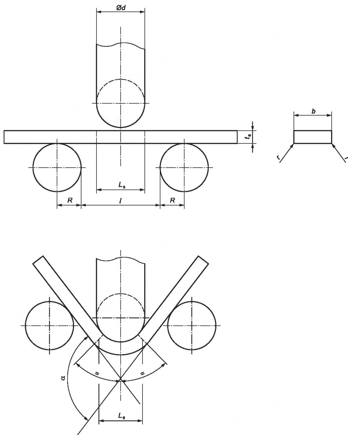
Рисунок 12 — Испытание на поперечный изгиб боковой стороны шва
