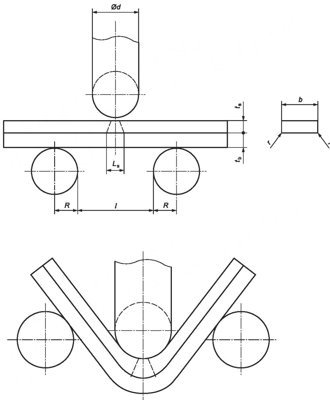
Рисунок 16 — Испытание на изгиб с опорной пластиной
