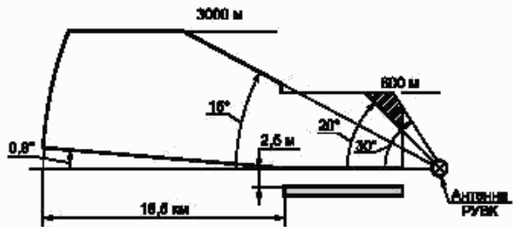
б) Зона наведения в вертикальной плоскости
