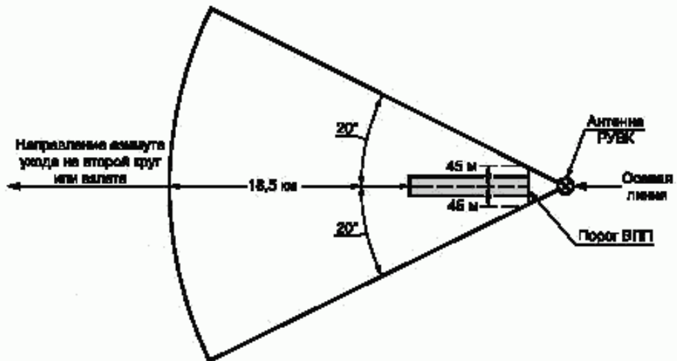
а) Зона наведения в горизонтальной плоскости
