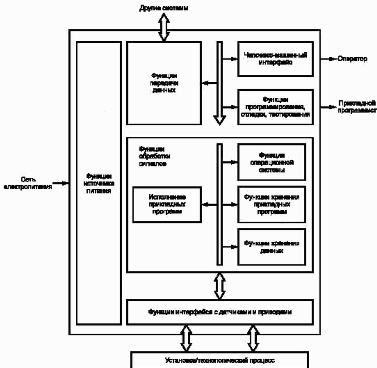
Рисунок 1 — Типовая функциональная структура конфигурации ПК
