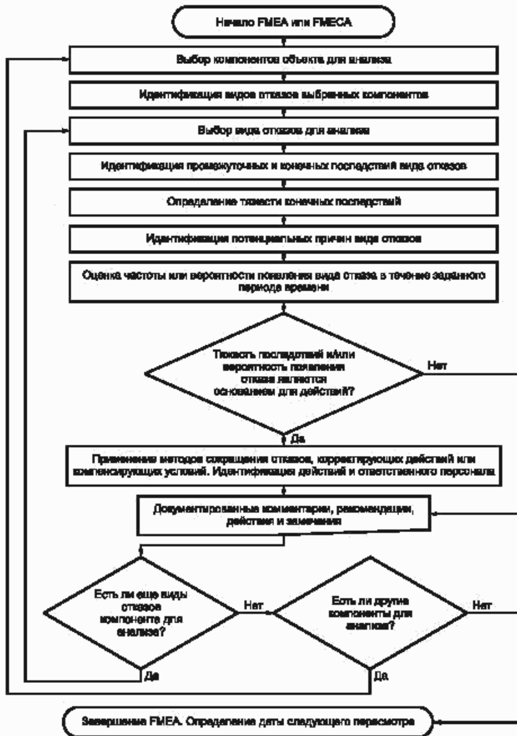
Рисунок 2 — Блок-схема анализа
