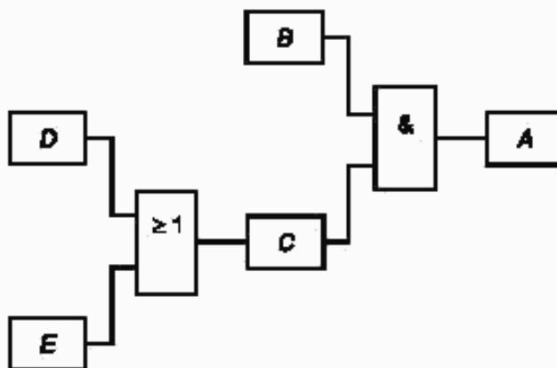
Рисунок 1 — Пример дерева неисправностей
