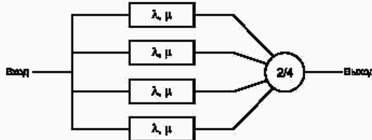
Рисунок 13 — Структурная схема надежности параллельной системы 2/4
