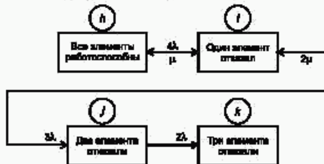
Рисунок 13 — Структурная схема надежности параллельной системы 2/4
