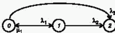
Рисунок 6 — Диаграмма состояний и переходов для системы, изображенной на рисунке 4, когда возможен прямой путь отказа из состояния 0 в состояние 2
