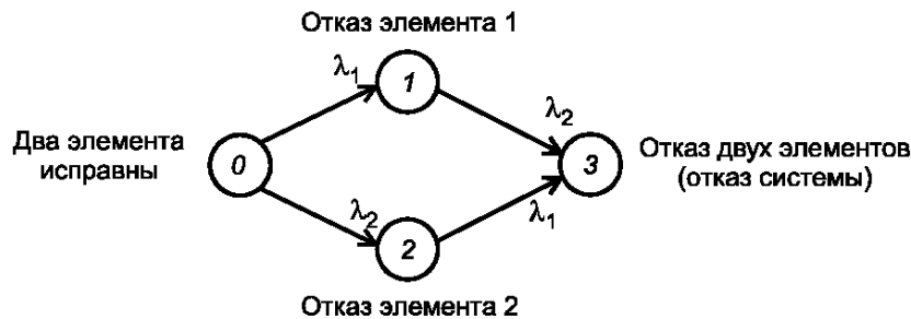
Рисунок 8 — Диаграмма состояний и переходов для системы с двумя восстанавливаемыми элементами
