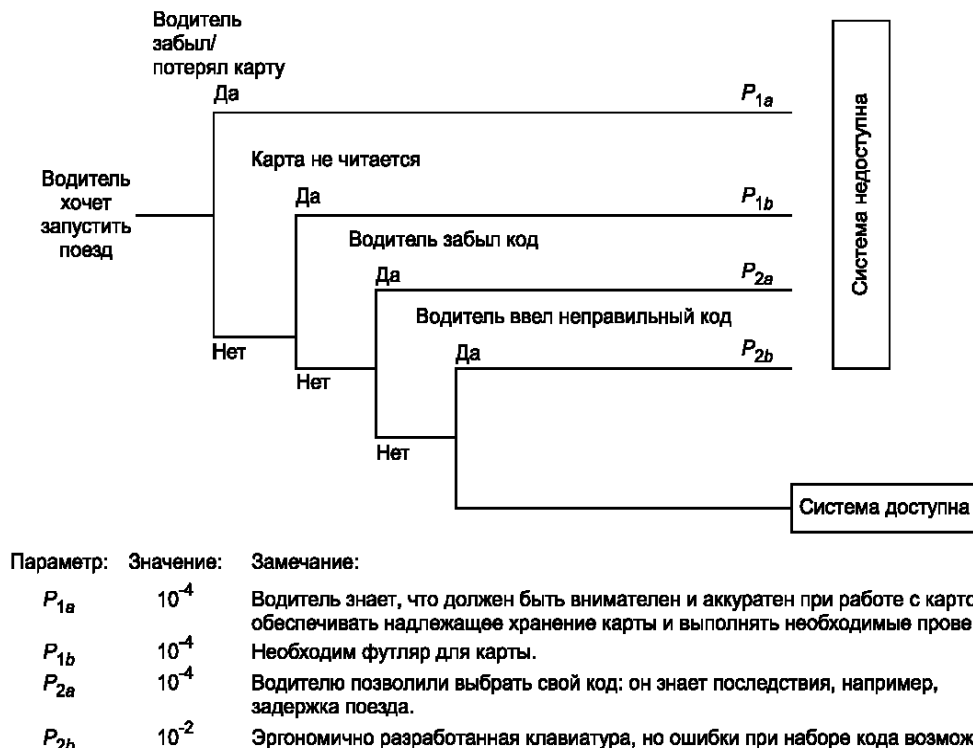
Рисунок А.11 — Человеческие ошибки, изображенные в виде дерева событий
