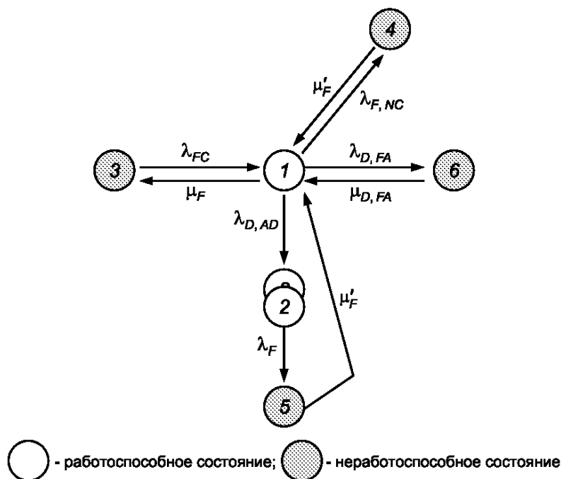
Рисунок А.7 — Диаграмма состояний и переходов
