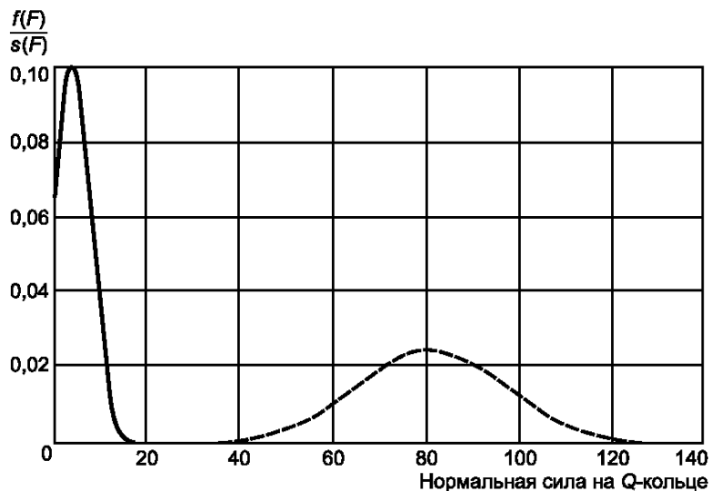
Рисунок А.12 — Пример применения критерия прочности напряжений
