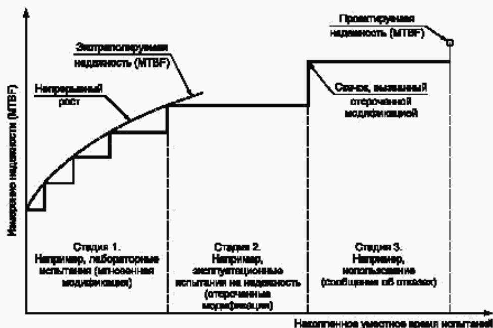
Рисунок 10 — Примеры кривых повышения надежности и скачков
