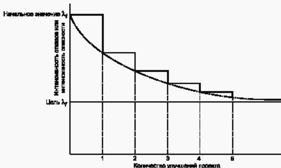
Рисунок 2 — Запланированное улучшение (снижение) эквивалентной интенсивности отказов
