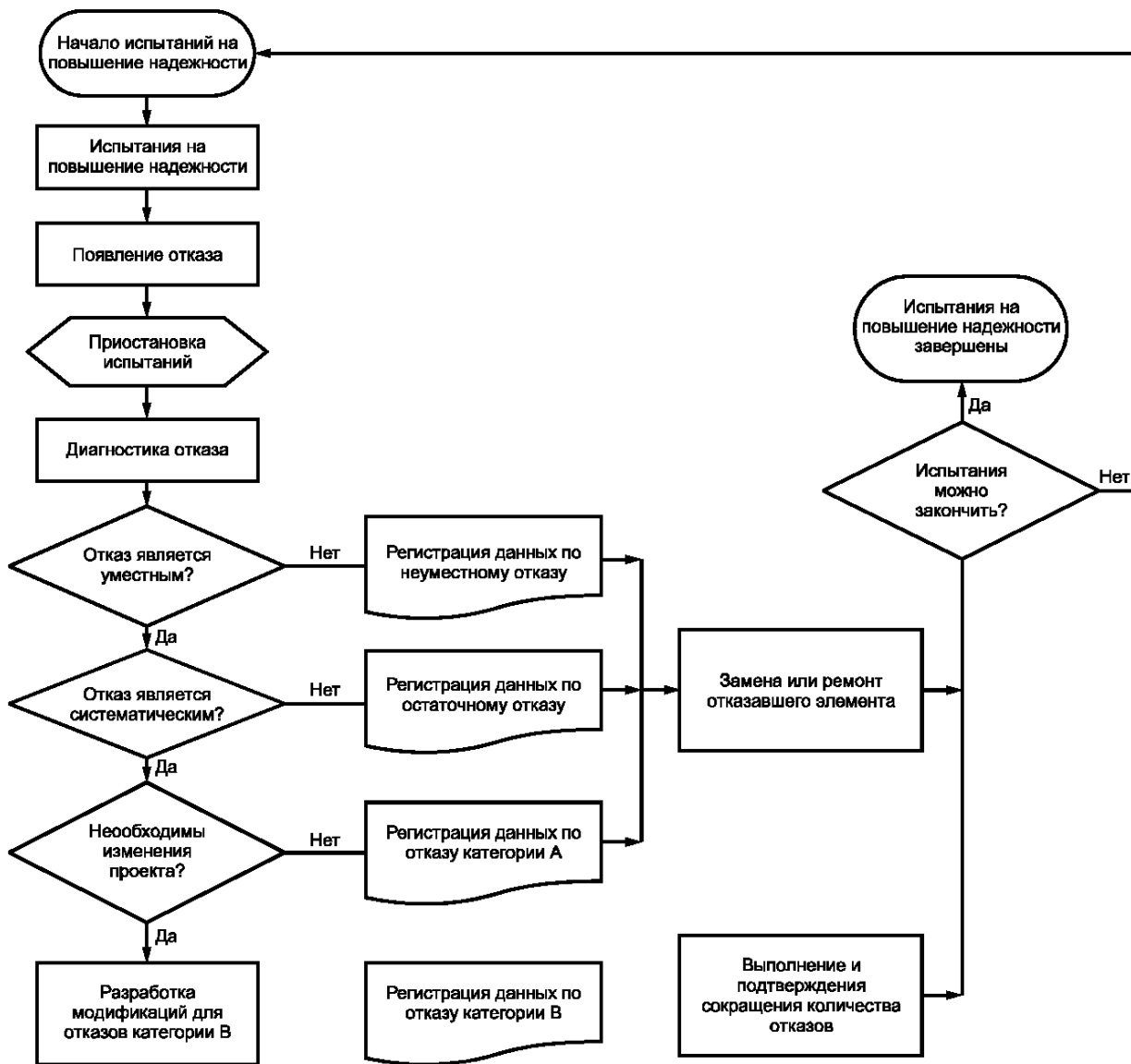
Рисунок 8 — Процесс испытаний на повышение надежности
