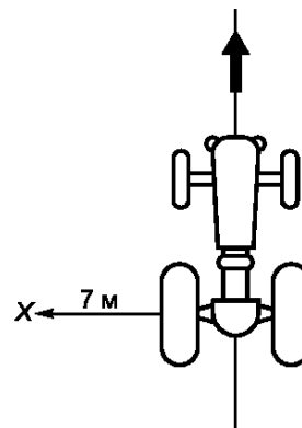
X — микрофон
