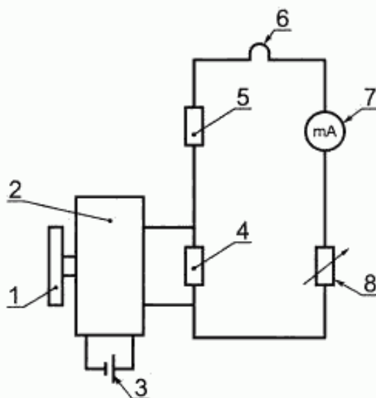
Схема потенциометра
