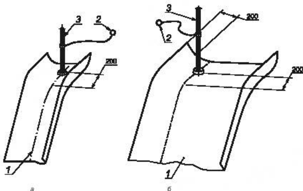
Рисунок Г.10 — Размещение испытательного устройства на горке
