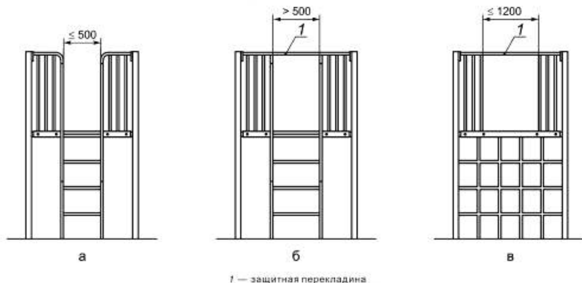
Рисунок 8 — Проемы в ограждениях
