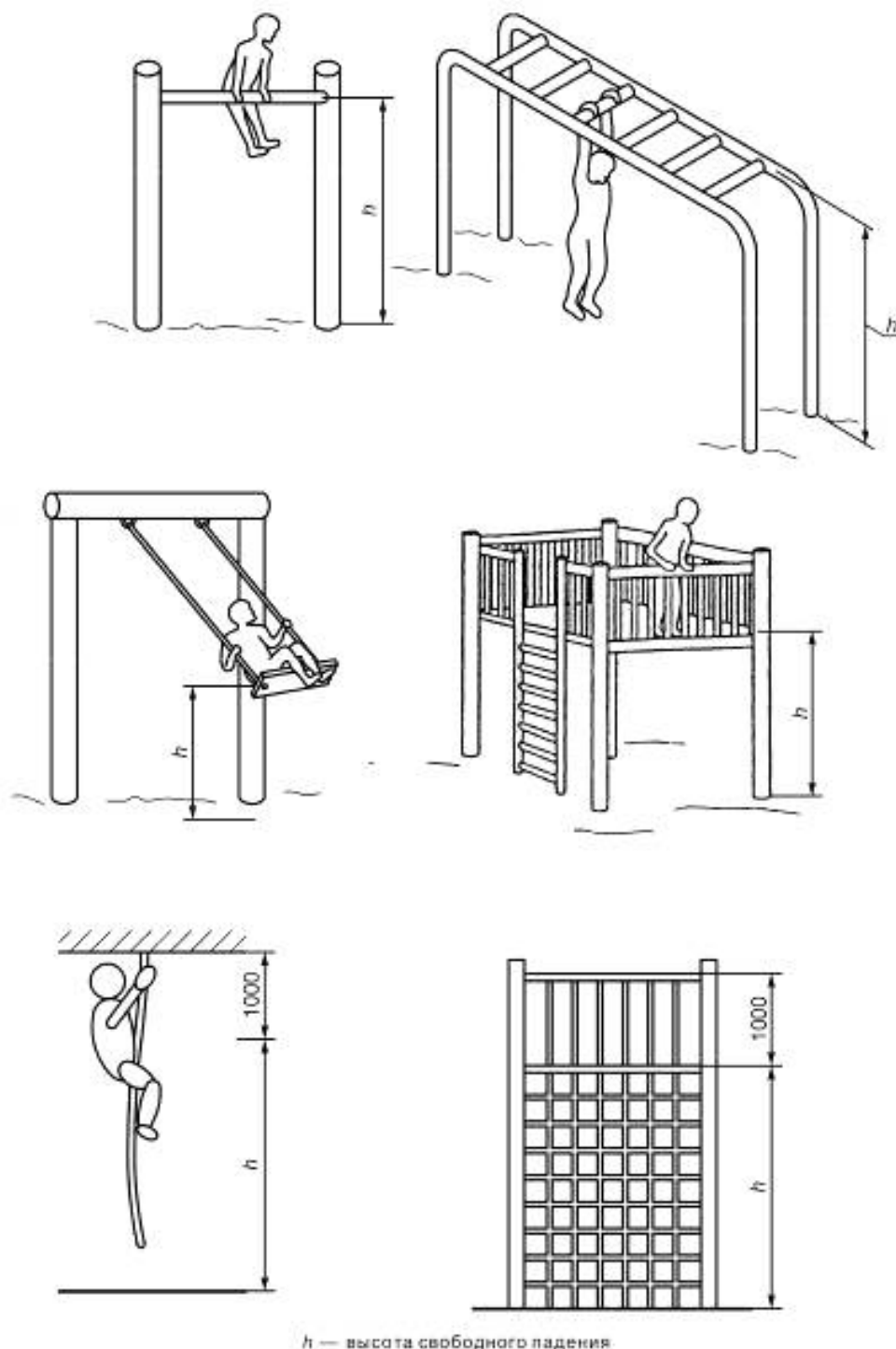
Рисунок 11 — Высота свободного падения h для различного оборудования
