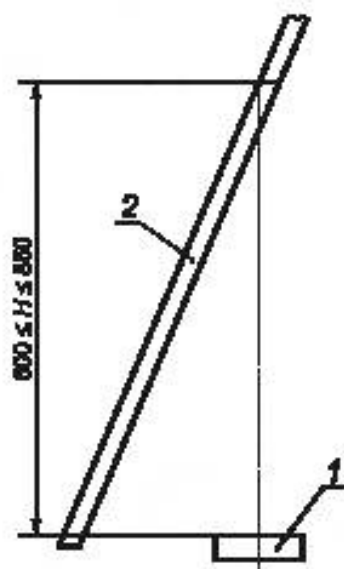
Рисунок 7 — Перила для лестниц
