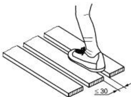
Рисунок 10 — Ширина зазоров на поверхностях наклоном до 45^\circ
