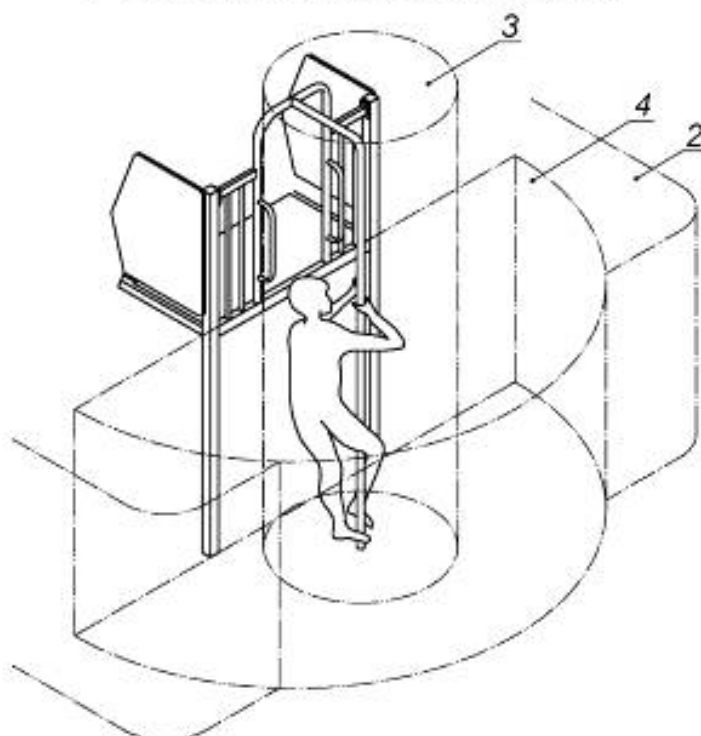
б — Зона падения и зона безопасности шеста
