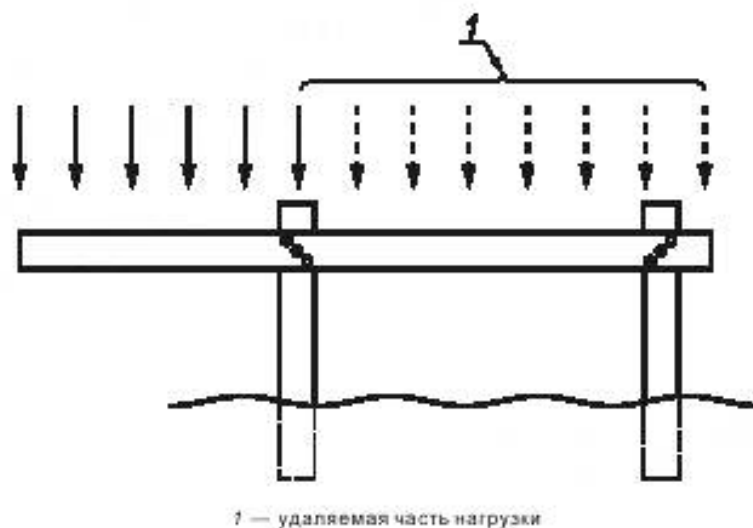
Рисунок 5 — Удаление части нагрузки
