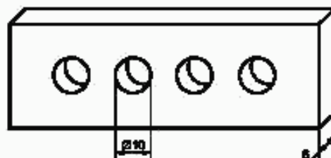
Рисунок 2 — Форма для образцов при испытании на текучесть
