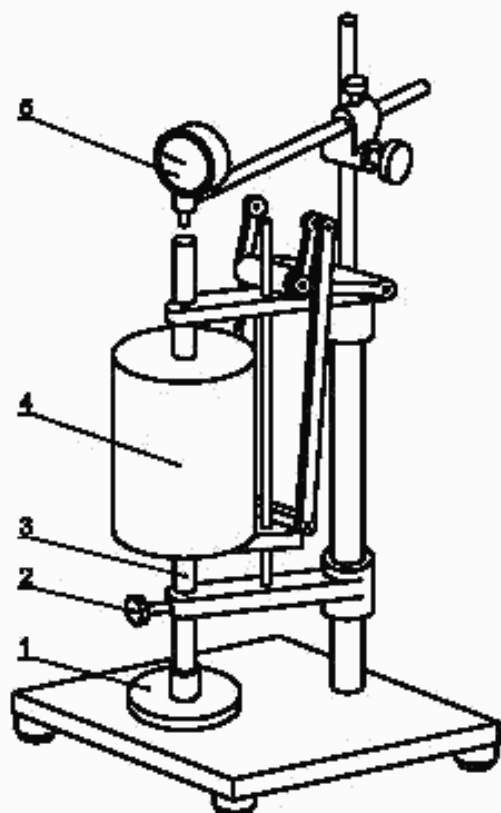
1 — латунная пластина; 2 — опорный винт; 3 — вал; 4 — металлический цилиндр; 5 — датчик
