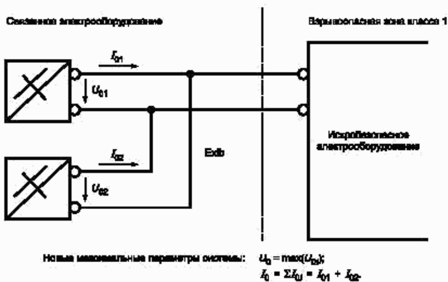
Рисунок В.2 — Параллельное соединение. Суммирование токов
