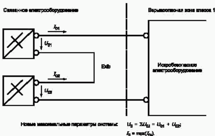
Рисунок В.1 — Последовательное соединение. Суммирование напряжений
