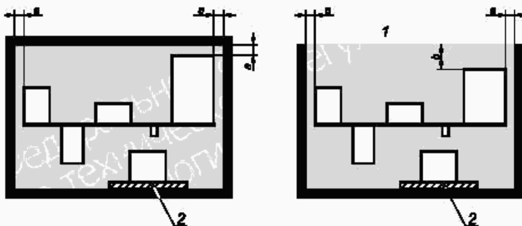
1 — наружная поверхность; 2 — твердый изоляционный материал (см. 7.2.3.2)
