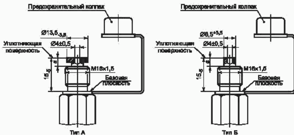
Рисунок А.2 — Присоединительные размеры клапанов контрольного вывода
