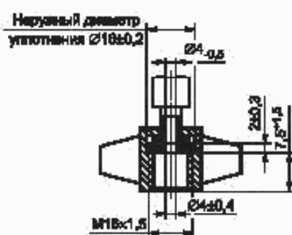
Рисунок А.1 — Наконечник для присоединения контрольных устройств к клапану контрольного вывода
