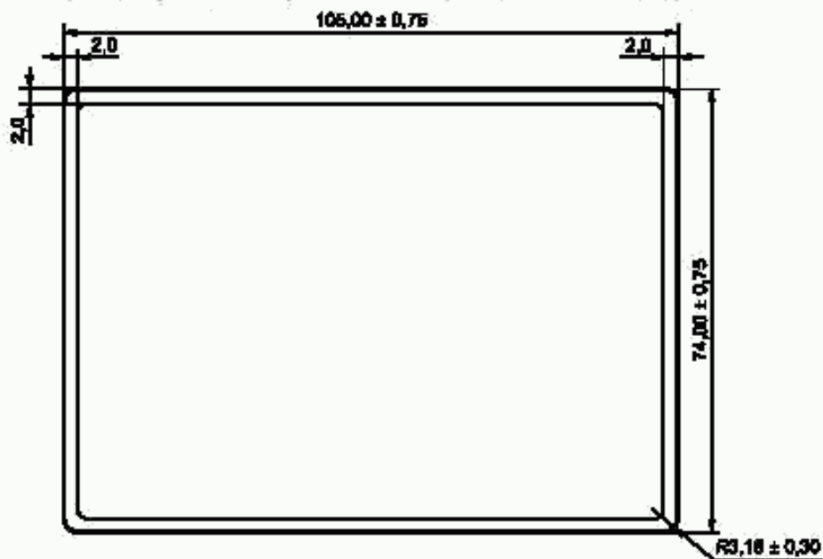
Рисунок 5 — Размеры и допуски документа ПД-2
