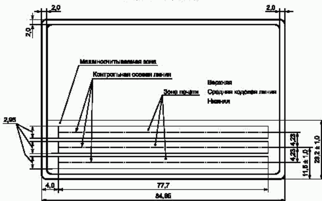
Рисунок 7 — Расположение и размеры МСЗ для документов типа ПД-1
