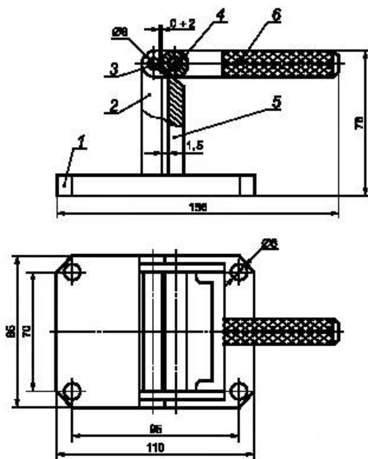
1 — плита; 2 — стойка; 3 — палец; 4 — обойма; 5 — упор; 6 — рукоятка
