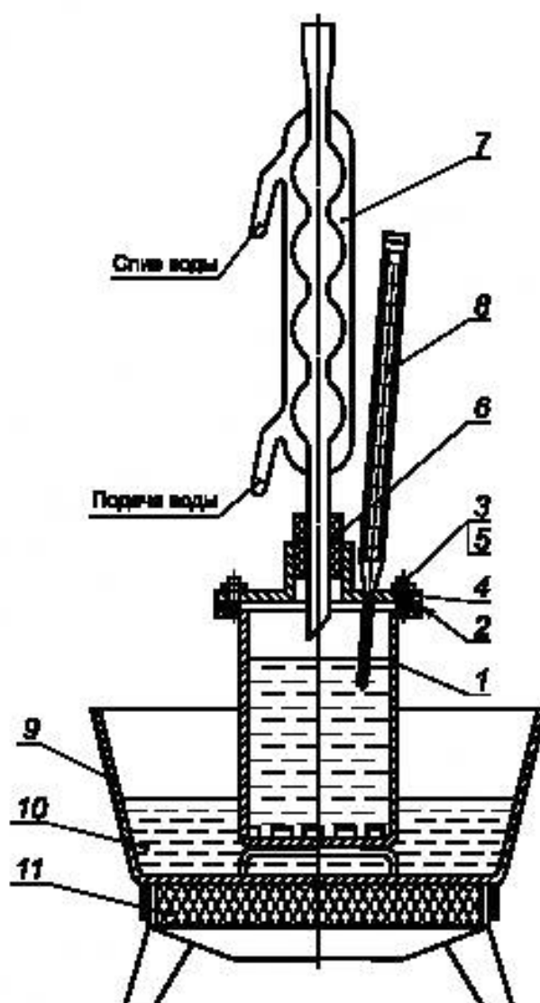
1 — стакан; 2 — прокладка резиновая; 3 — гайка; 4 — крышка; 5 — шпилька; 6 — резиновая пробка; 7 — шариковый холодильник; 8 — термометр; 9 — ванна; 10 — глицерин (вода); 11 — плита
