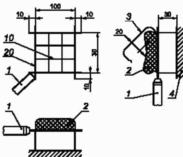
Рисунок А.1 — Рамка для закрепления ватного тампона
