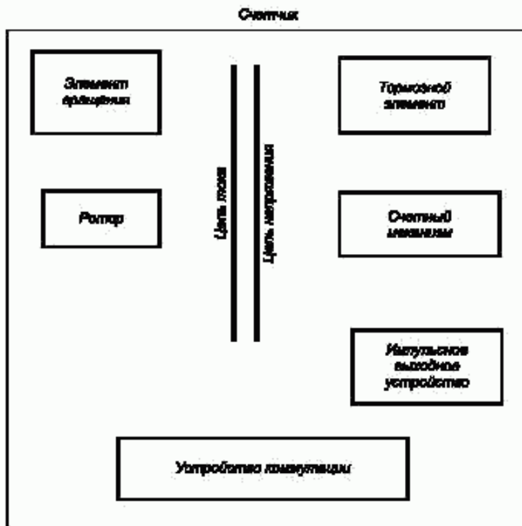
Рисунок С.1 — Структурная схема электромеханического счетчика
