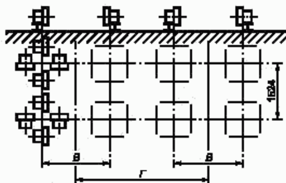
Рисунок Г.3 — Трансформаторы массой от 255 до 300 т
