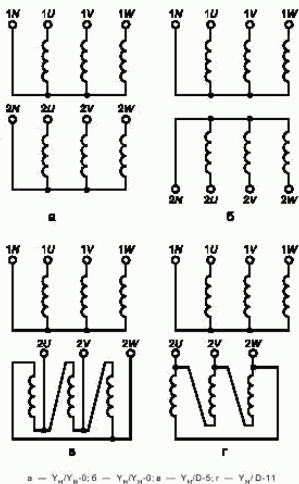
Рисунок Ж.4 — Маркировка трехфазных двухобмоточных трансформаторов
