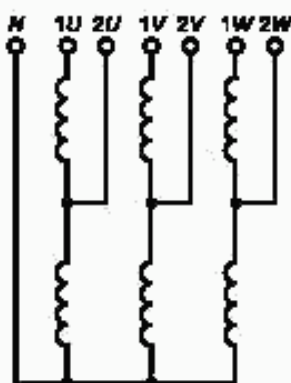
Рисунок Ж.7 — Маркировка трехфазного автотрансформатора ( Y_H авто/D-0)
