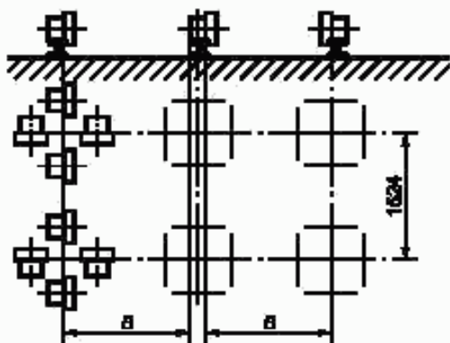
Рисунок Г.2 — Трансформаторы массой от 200 до 255 т
