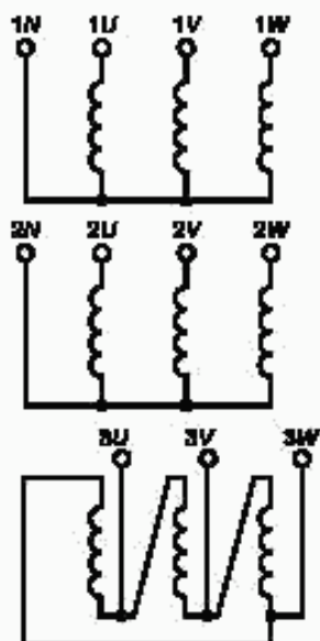
Рисунок Ж.5 — Маркировка трехфазного трехобмоточного трансформатора ( Y_H/Y_H/D-0-5 )
