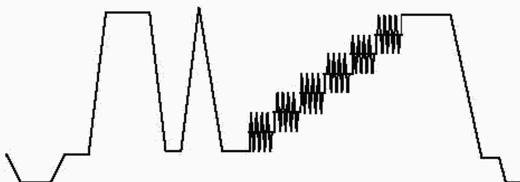
Рисунок 2 — Графическое изображение измерительного сигнала, содержащего сигнал Н1
