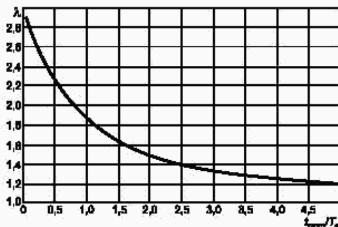
Рисунок В.1 — Зависимость коэффициента \lambda от t_{\text{откл}}/T_a
