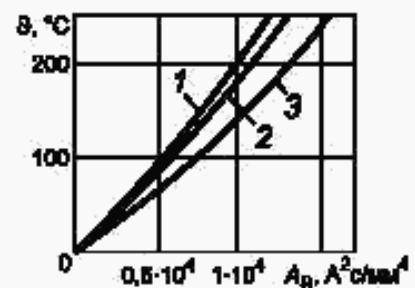
Материалы проводов: 1 — сплавы АЖ и АЖКП; 2 — сплавы АН и АНКП; 3 — алюминий марок А, АКП, АпКП и сталеалюминий марок АС, АСКП, АСКС, АСК, АлС, АпСКС, АлСК
