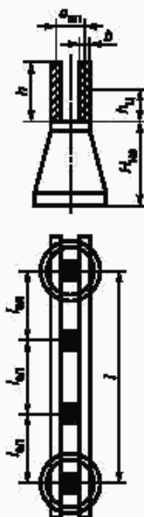
Рисунок 4 — Двухполосная шина
