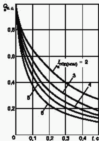
Рисунок 18 — Кривые для определения Q_{к.д} от асинхронного электродвигателя
