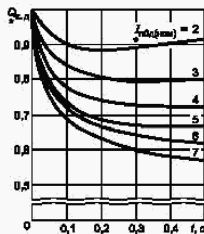
Рисунок 16 — Кривые для определения Q_{к.д} от синхронного электродвигателя
