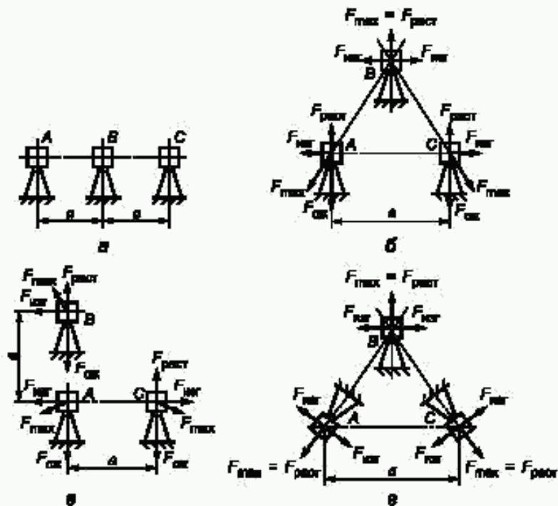
Рисунок 2 — Схемы взаимного расположения шинных конструкций
