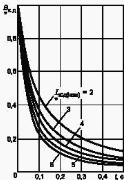
Рисунок 17 — Кривые для определения I_{к.д} от асинхронного электродвигателя
