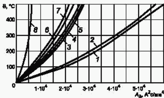
Материалы проводников: 1 — ММ; 2 — МТ; 3 — АМ; 4 — АТ; 5 — АДО, АСТ; 6 — АД31Т1; 7 — АД31Т; 8 — СгЗ
