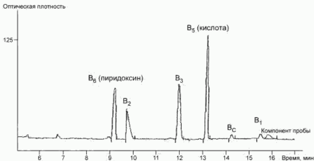
Рисунок Б.3 — Электрофореграмма экстракта премикса
