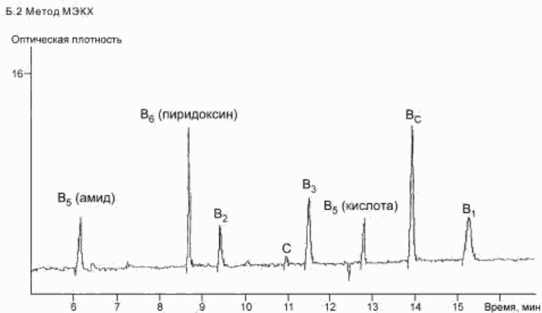
Рисунок. Б.2 — Электрофореграмма градуировочного раствора
