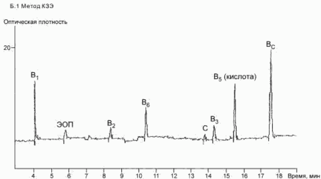
Рисунок. Б.1 — Электрофореграмма градуировочного раствора
