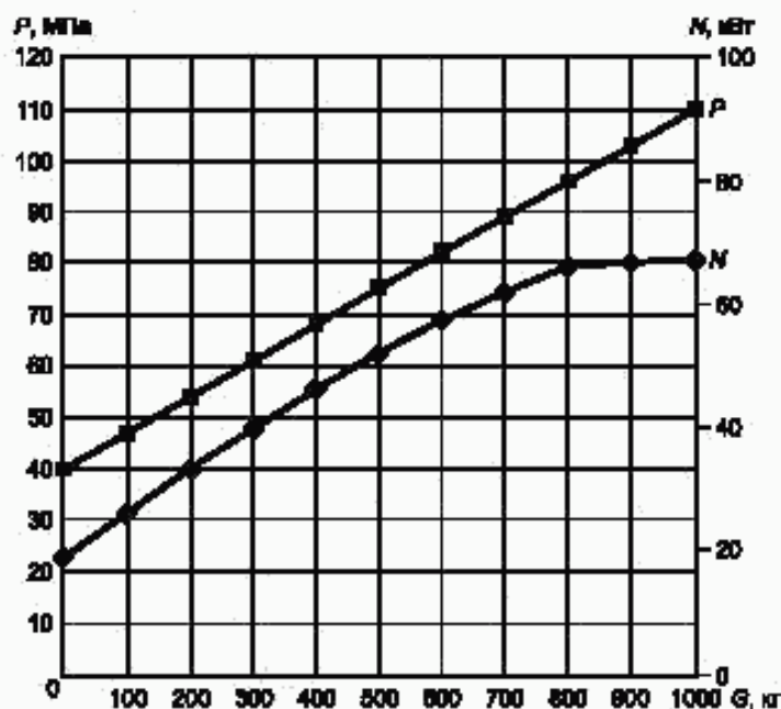
Рисунок 1 — Графическое изображение нагрузочной характеристики гидросистемы
