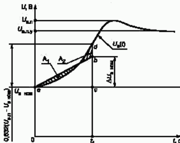
Рисунок А.1 — Определение номинальной скорости нарастания напряжения возбуждения
