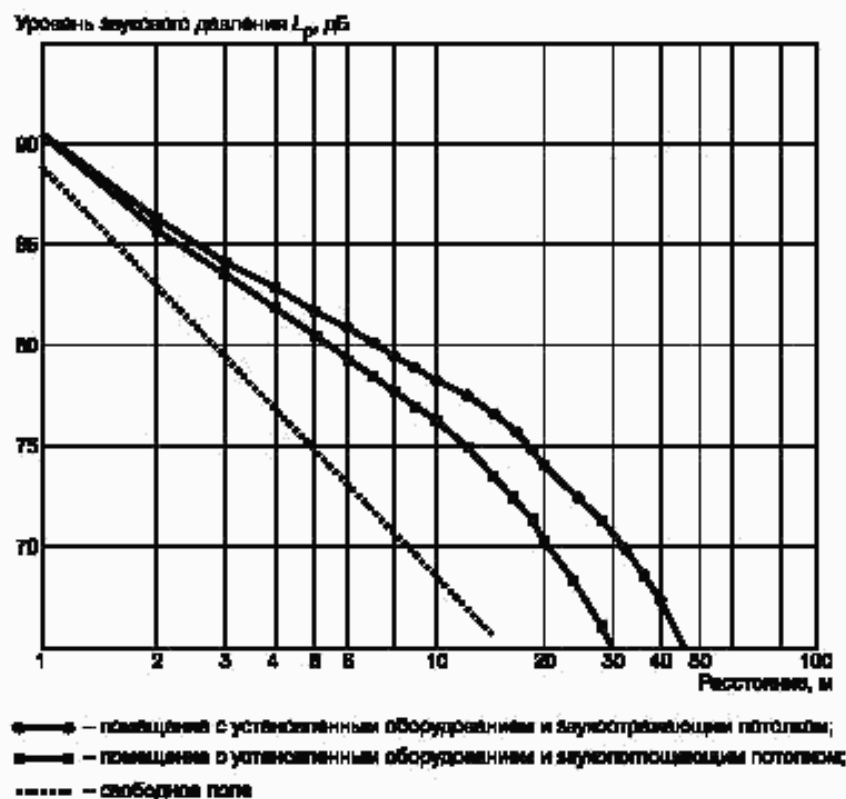
Рисунок 2 — Типичные линии пространственного распределения звука, излученного ненаправленным точечным источником звуковой мощностью 100 дБ в плоском заполненном оборудованном помещении со звукопоглощающим и со звукоотражающим потолком
