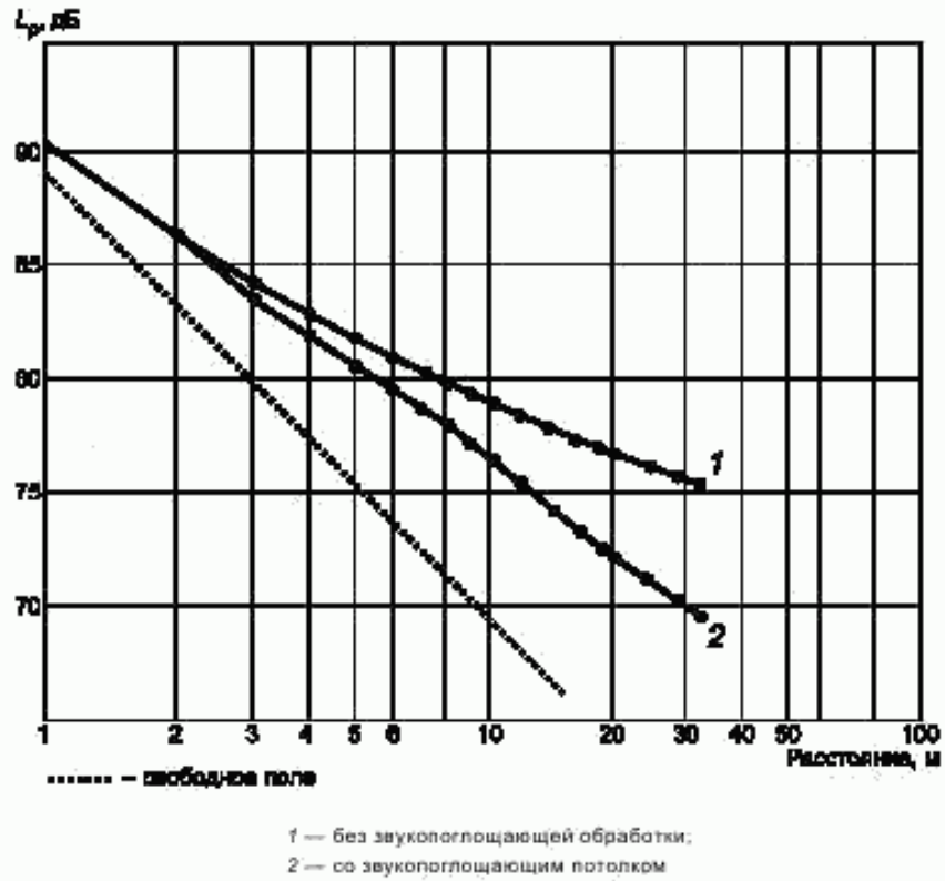
Рисунок D.1 — Рассчитанные линии пространственного распределения звука
