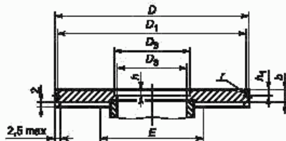
Рисунок 2 — Опорный фланец
