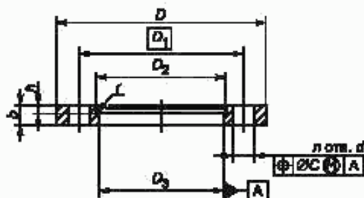
Рисунок 3 — Накладной фланец
