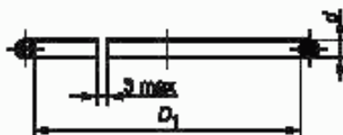
Рисунок 4 — Установочное кольцо
