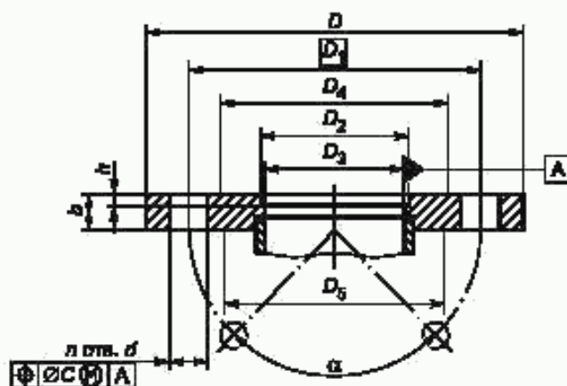
Рисунок 1 — Неподвижный фланец
