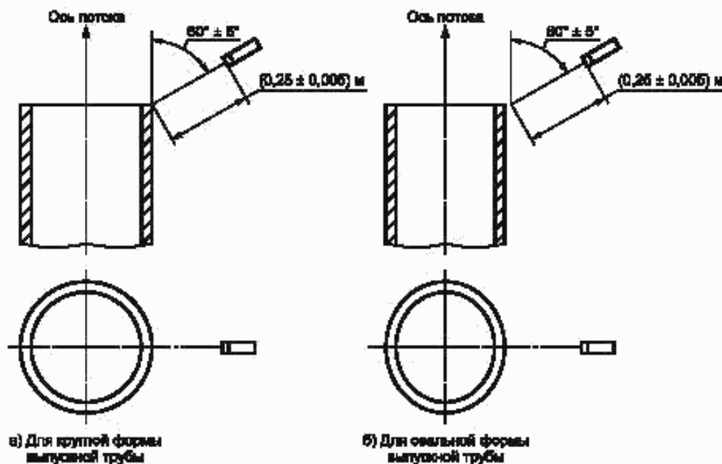
Рисунок 5 — Расположение микрофона для измерения шума процесса выпуска
