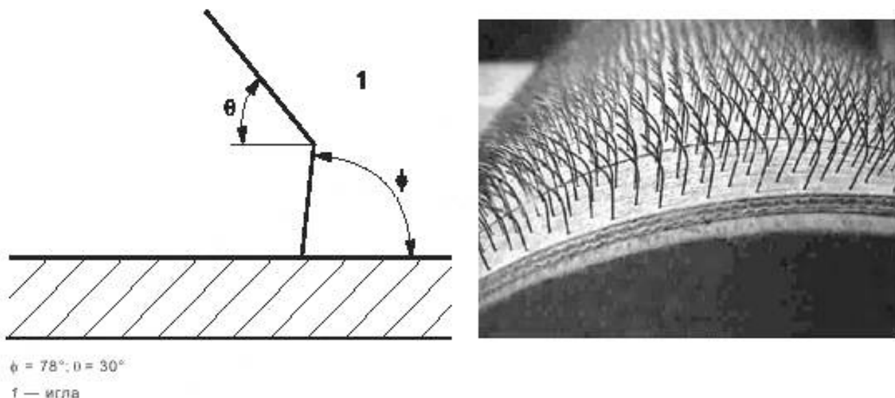
Рисунок 1 — Электромеханический разрыхлитель
