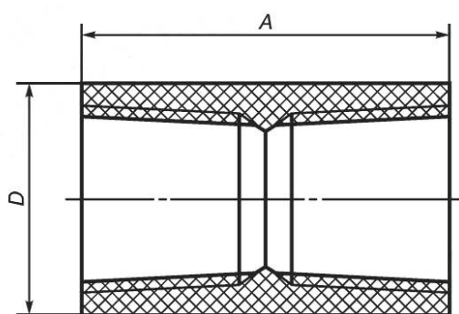
A — длина муфты; D — наружный диаметр
