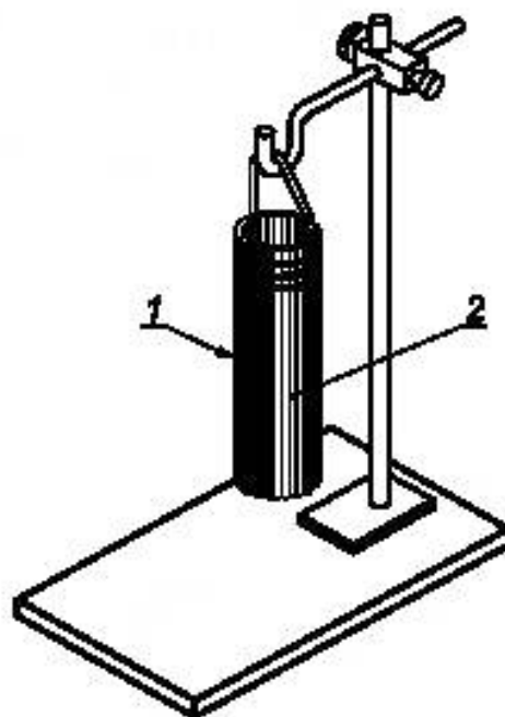
1 — изогнутый лист из негорючего материала; 2 — хлопковые фитили
