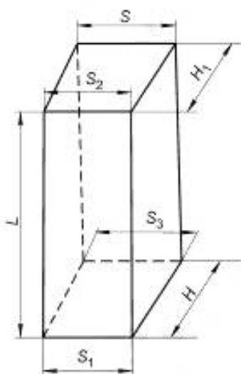
Рисунок 7 — Фасонное изделие номер 41
