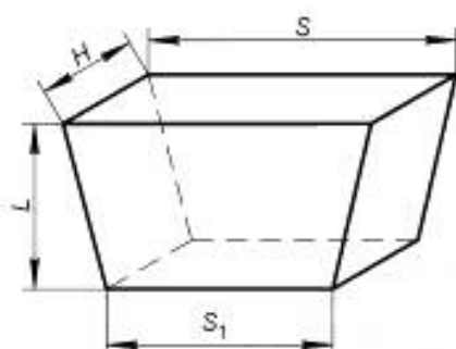
Рисунок 3 — Трапецидальный двусторонний клин номеров 6—21
