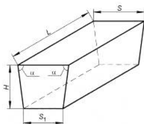
Рисунок 1 — Ребровый двусторонний клин
