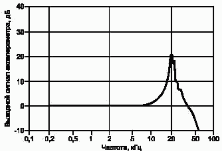
Рисунок 9 — Типичная частотная характеристика акселерометра на магните
