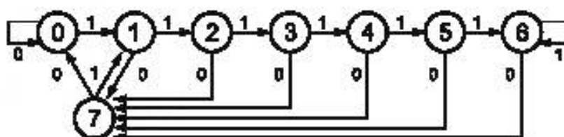
Рисунок Б.2 – Переходы состояний маскирования фреймов
