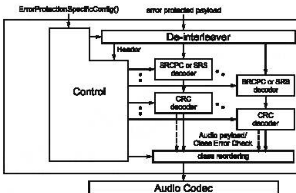
Рисунок 5 - Схема декодера EP
