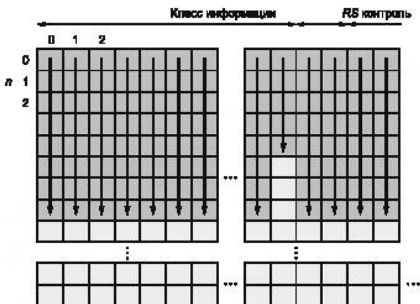
Рисунок 13 – Матрица чередования в случае RS класса
