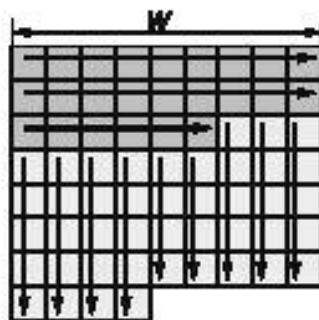
Рисунок 10 – Матрица чередования в непрямоугольном случае
