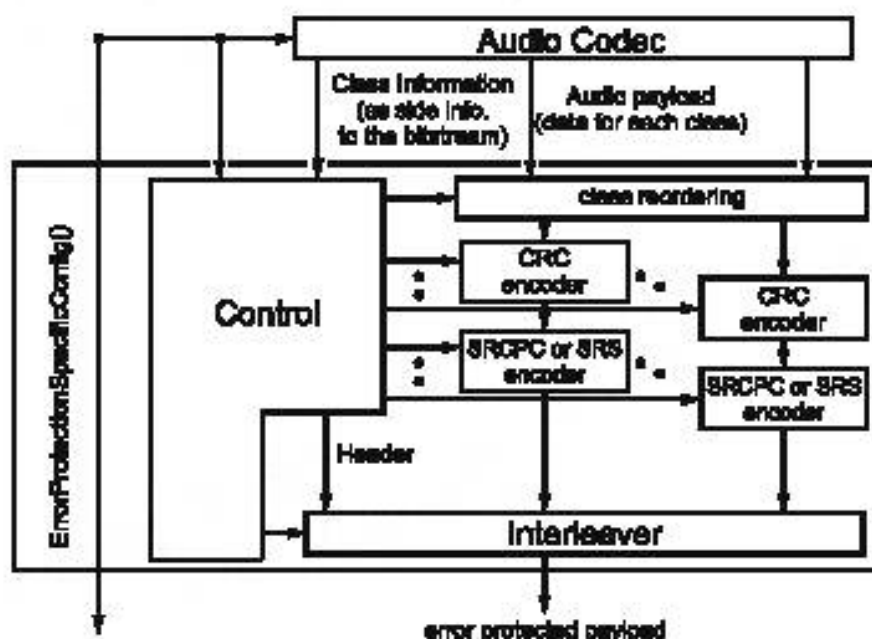
Рисунок 4 - Схема кодера EP
