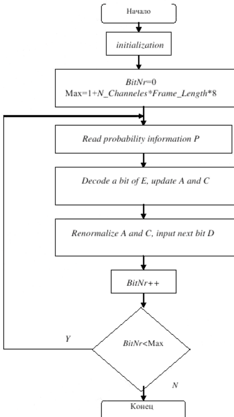
Рисунок 2 – Блок-схема арифметического декодера
