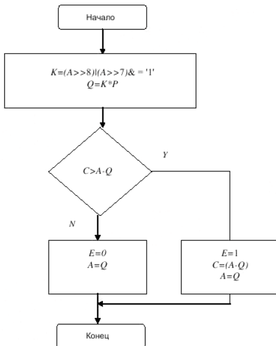
Рисунок 4 – Декодирование бита E , обновление A и C
