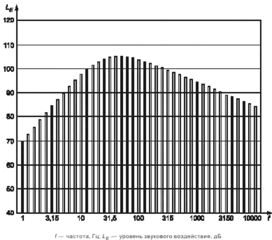
Рисунок А.1 — 1/3-октавный спектр Вебера ударной волны
