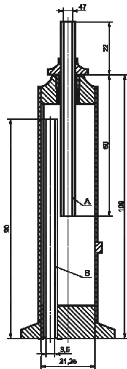
Рисунок А1.2 — Резервуар
