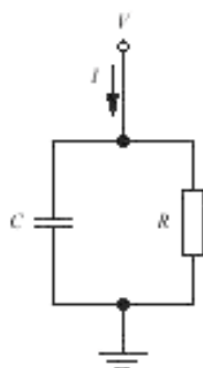
Рисунок 3 – Эквивалентная электрическая цепь заряжения проводника
