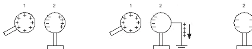
1а) – Сближение заряженного объекта (1) с незаряженным объектом (2)
