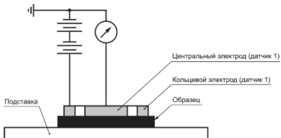
Рисунок 2 — Принцип подключения электродов для измерения поверхностного сопротивления
