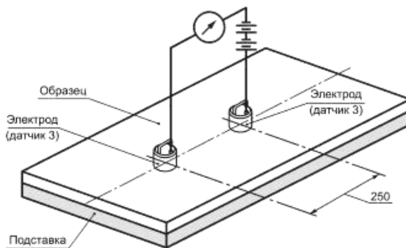
Рисунок 8 — Принцип измерения сопротивления от точки до точки
