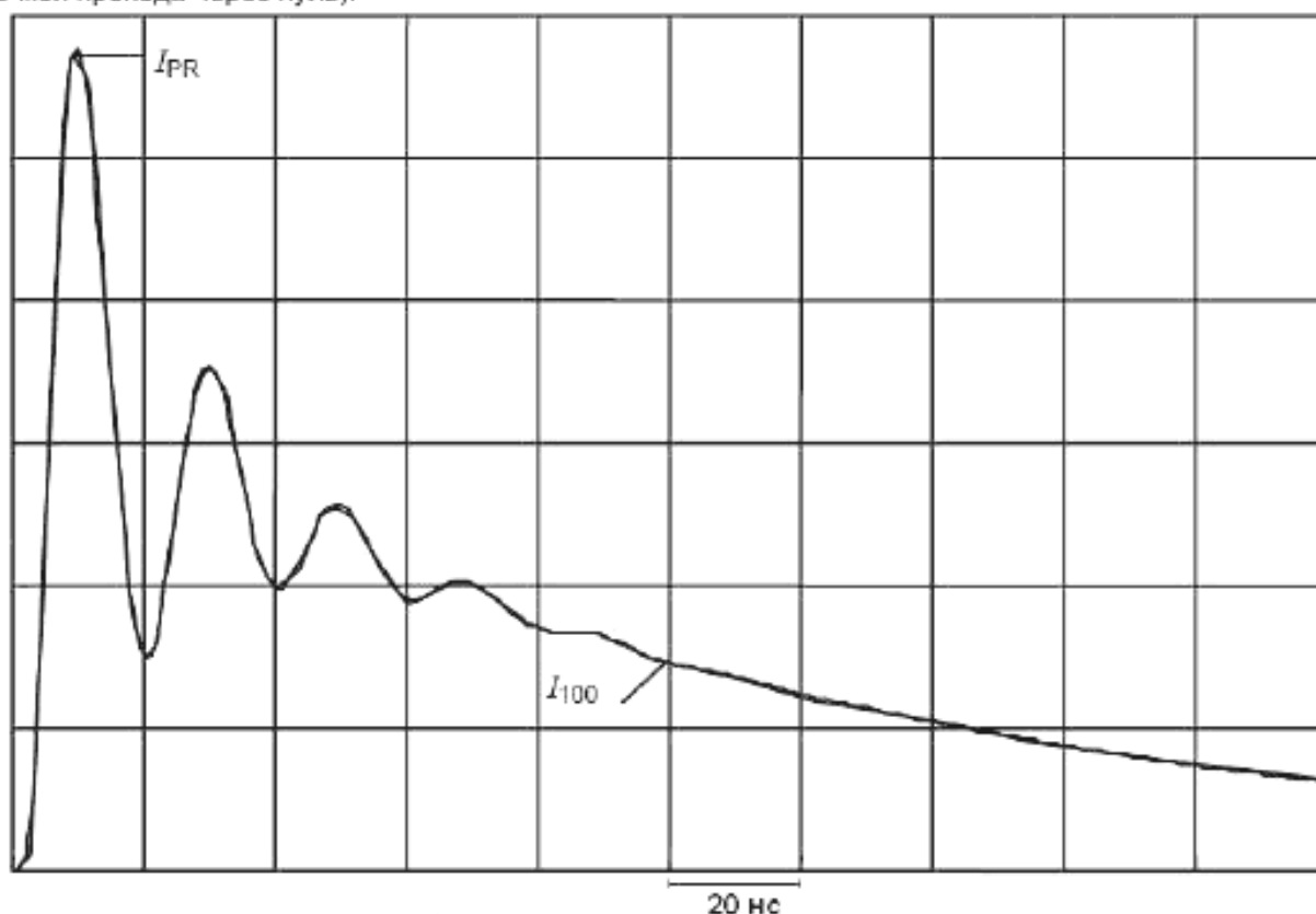
Рисунок 3 – Типичный импульс тока через резистор 500 Ом
