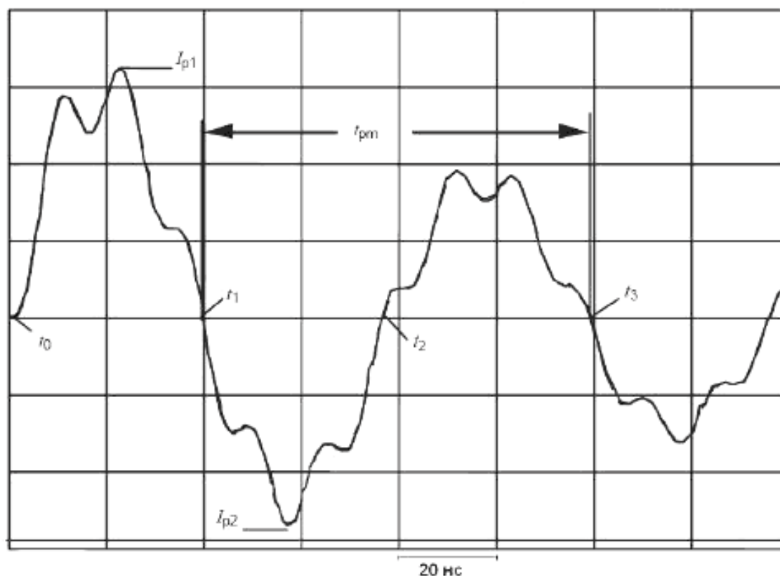
Рисунок 2 – Типичный импульс тока через закорачивающий провод
